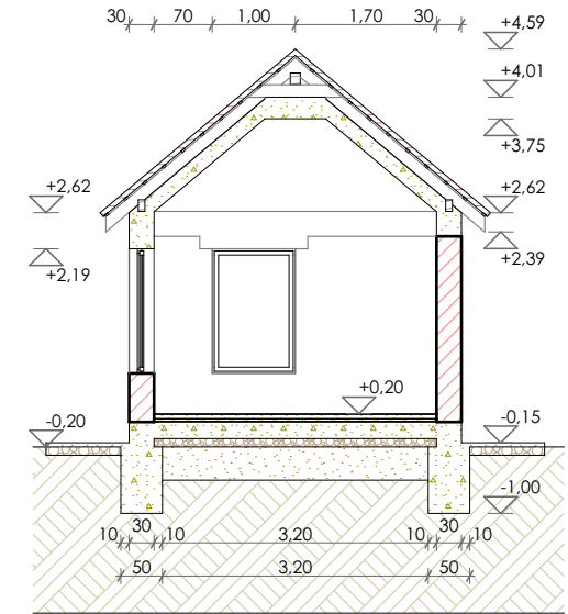
A-A Section
