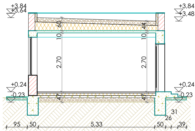
A-A Section
