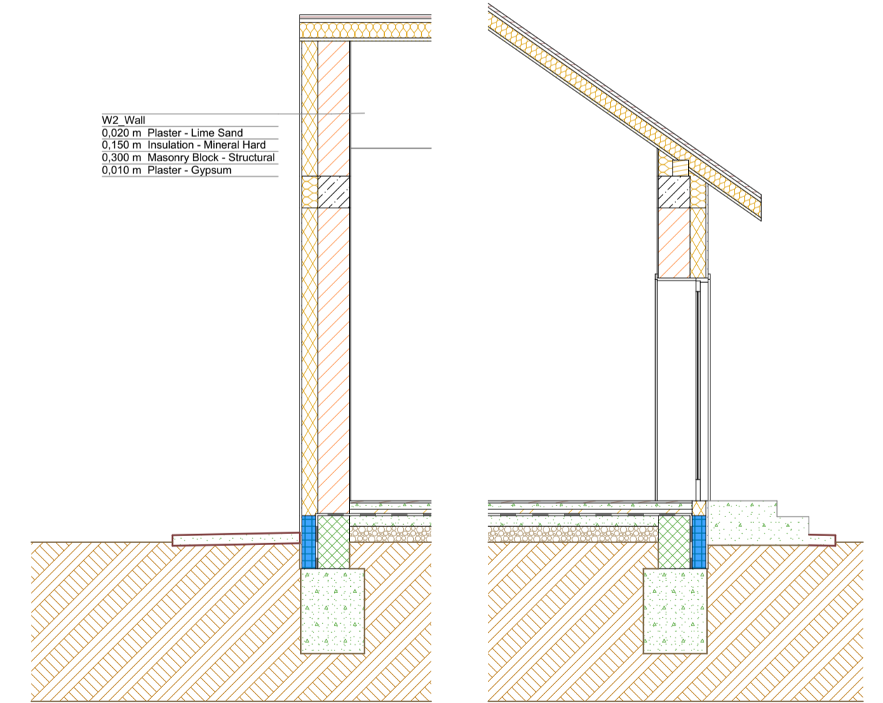
S-02 Section
