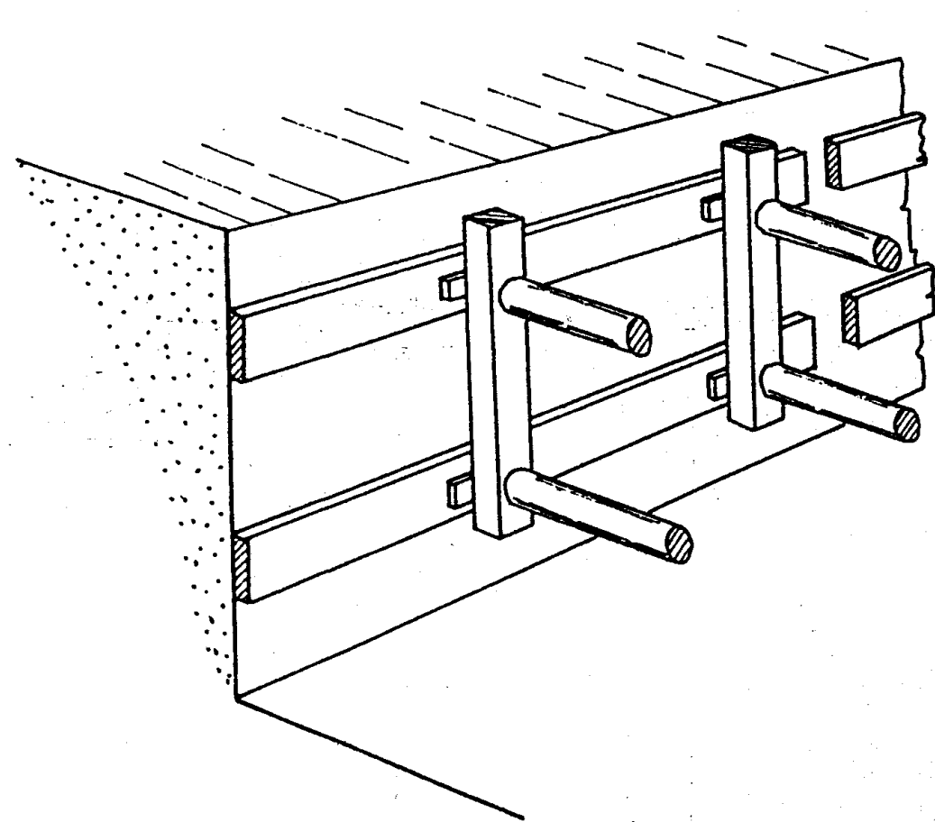
2.4. ábra Állított pallózási mód
