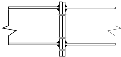
(e) Homloklemez gerendaillesztés
