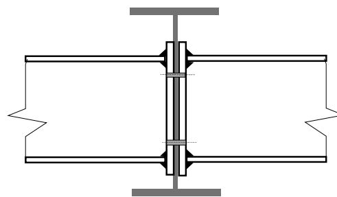
(h) Két gerenda–gerenda kapcsolat (kétoldali elrendezés)
