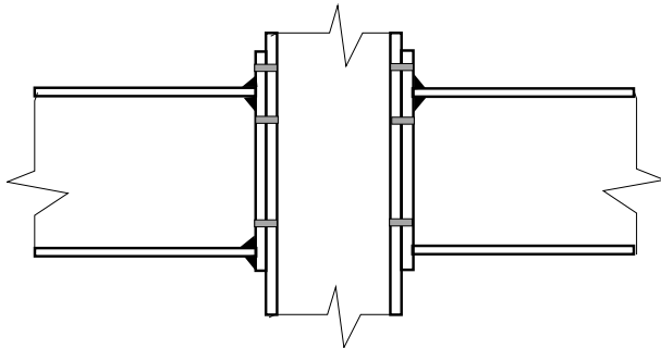
(c) Két túlnyúló homloklemez csavarozott kapcsolat (kétoldali elrendezés)
