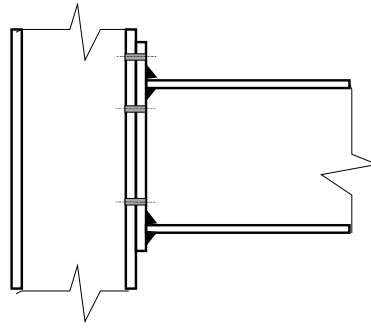
(b) Túlnyúló homloklemez csavarozott kapcsolat
