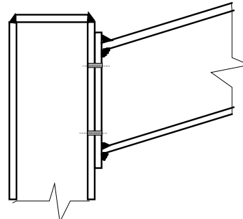
(d) Nem túlnyúló homloklemez csavarozott kapcsolat
