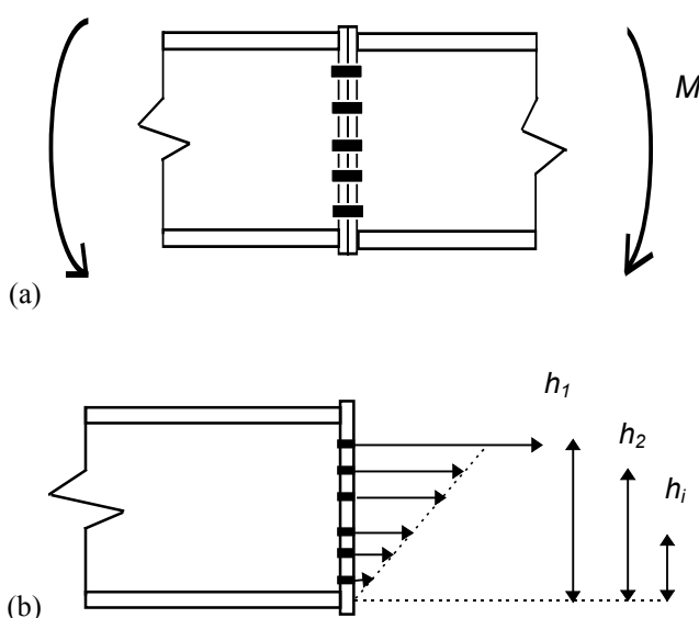
A.21.16. ábra: Vékony homloklemezrel kialakított kapcsolat. (a) Elrendezés; (b) A belső erők megoszlása a terhelés kezdetén
