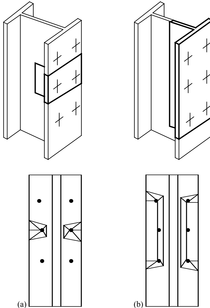
A.21.19. ábra: Képlékeny mechanizmusok: (a) egyedi; (b) csoportos mechanizmus
