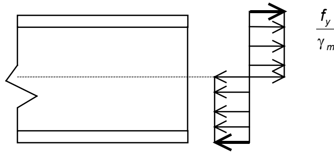
A.21.9. ábra: A keresztmetszet képlékeny tervezési nyomatóki ellenállásához tartozó belső erők (itt: feszültségek)
