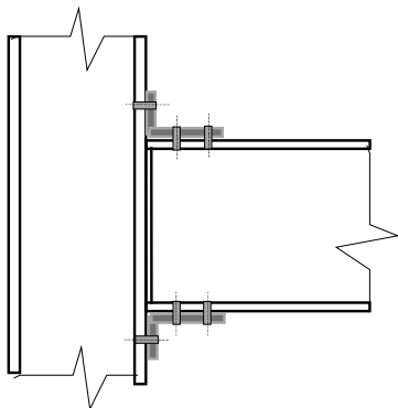
(g) Övbekötő szögacélos csavarozott kapcsolat
