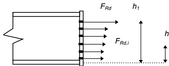
A.21.17. ábra: A belső erők képlékeny megoszlása
