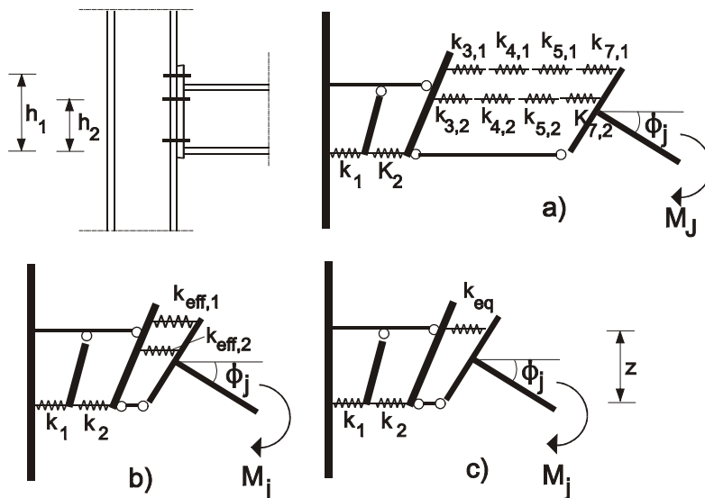
A.21.12. ábra: Egynél több húzott csavarsorral rendelkező homloklemez-eszlop-gerenda kapcsolatok rugómodellje
