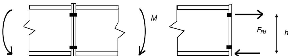
A.21.13. ábra: Egy húzott csavarsorral rendelkező kapcsolat
