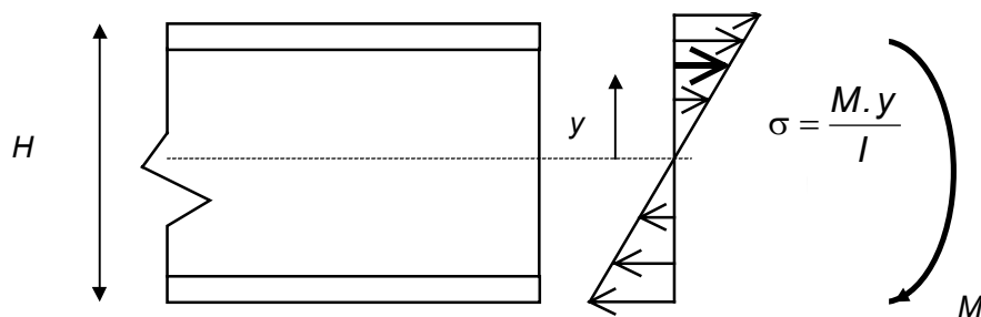
A.21.7. ábra: A belső erők (itt: feszültségek) rugalmas megoszlása hajlított gerenda-keresztmetszetben ( I az inercianyomatékot jelöli). (a) gerenda; (b) belső feszültségek; (c) külső erő
