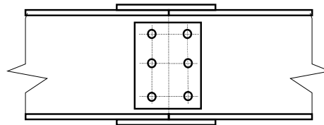
(f) Hevederlemez gerendaillesztés
