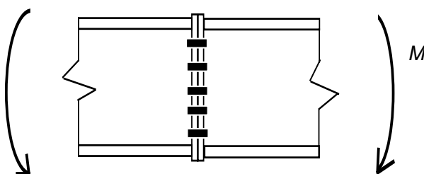
A.21.14. ábra: Egynél több húzott csavarsorral rendelkező kapcsolat
