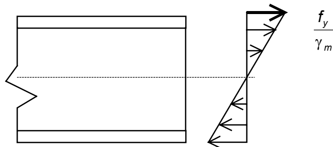
A.21.8. ábra: A keresztmetszet legnagyobb rugalmas tervezési nyomatéki ellenállásához tartozó belső erők (itt: feszültségek)
