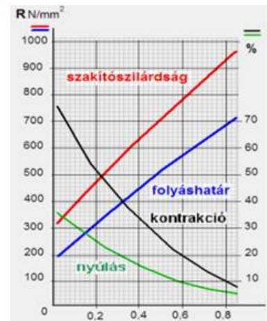
Széntartalom hatása
