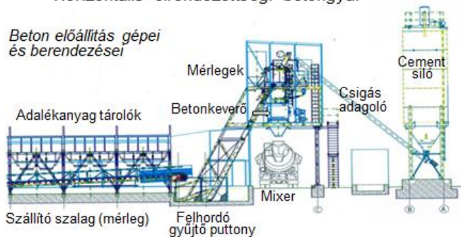
Horizontális elrendeztségi betongyár
