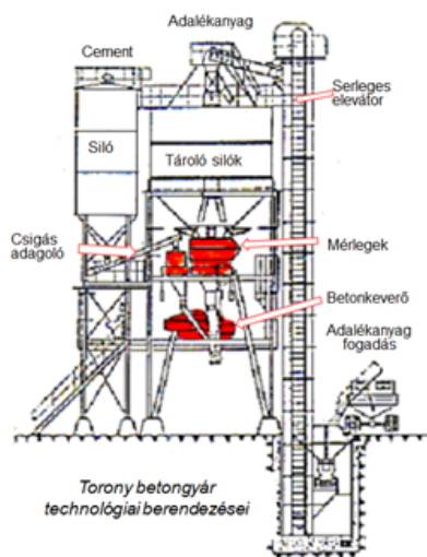
Vertikális betongyár
