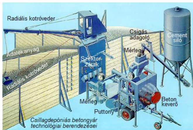
Horizontális elrendeztségi betongyár
