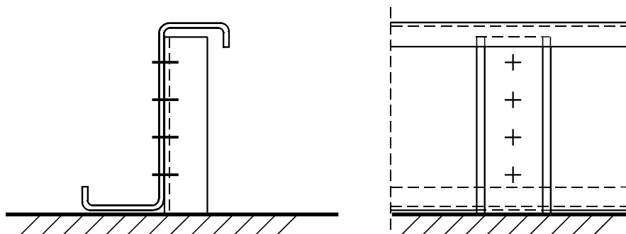
3.1 ábra: vékonyfalú gerendák tipikus megtámasztása
