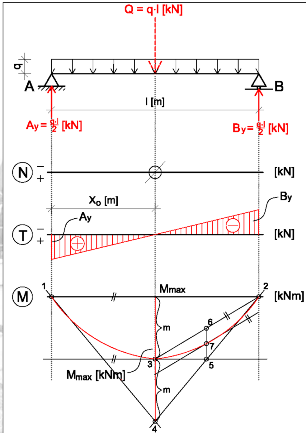
7. ábra. Egyenletesen megoszló teherrel terhelt kéttámaszú tartó [Szabó I. G. 2012]
