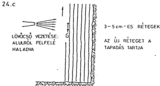
24. ábra: VASTAG LÖVTETON RÉTEGEK KÉSZÍTÉSE
