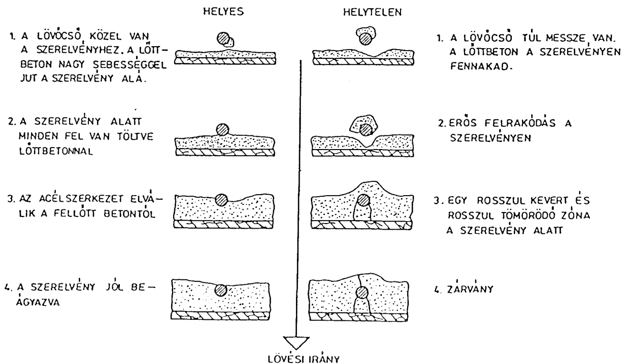
23. ábra: LÖVŐCSŐ HELYES ÉS HELYTELEN KEZELÉSE
