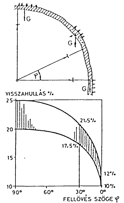
21.d ábra: LÖVÉSI IRÁNY HATÁSA
