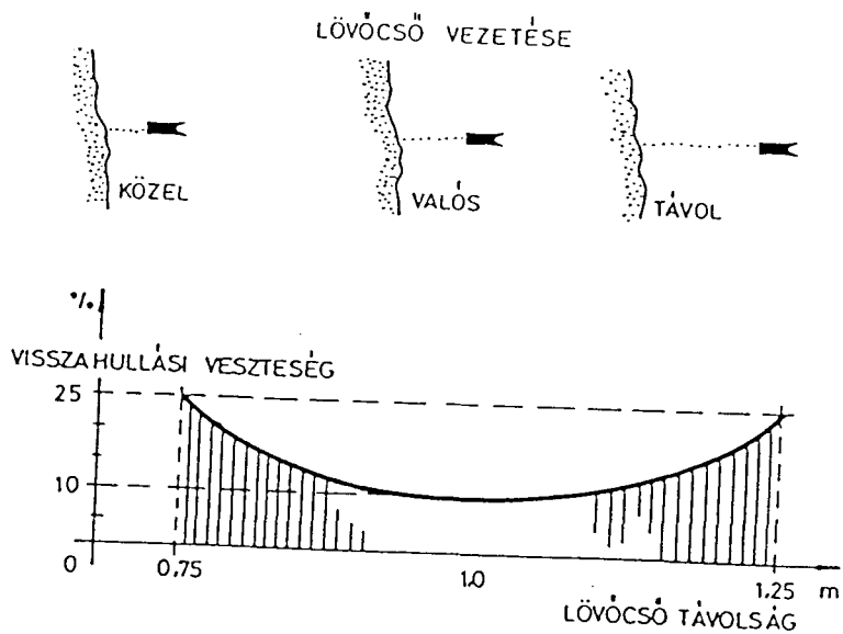
21.c ábra: LÖVÉSI TÁVOLSÁG HATÁSA
