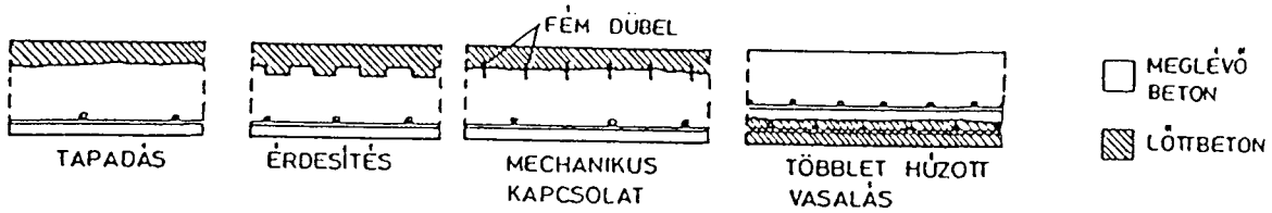
31. ábra: SÍKLEMEZFÖDÉM MEGERŐSÍTÉSE
