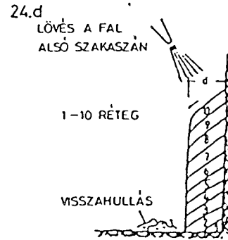
24. ábra: VASTAG LÖVTETON RÉTEGEK KÉSZÍTÉSE
