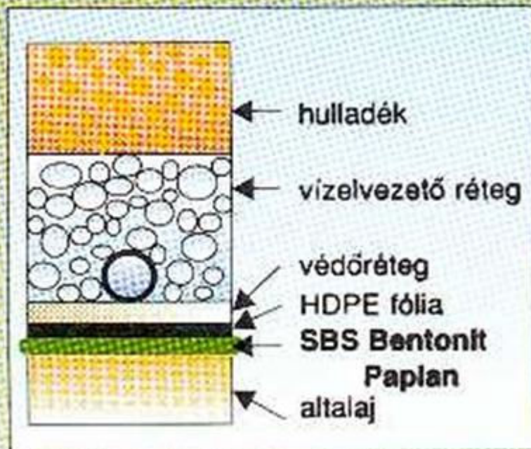
Hulladéklerakó alsó szigetelés
