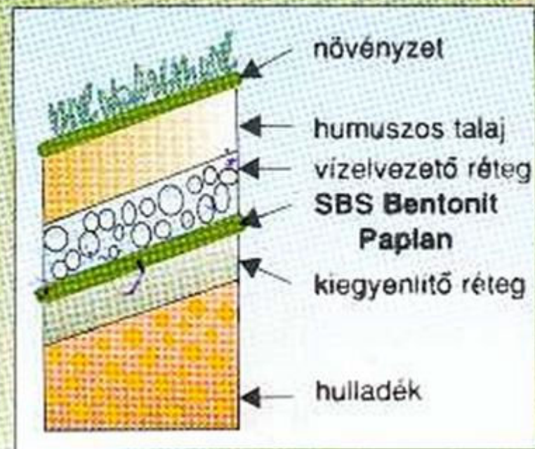
Felső réteg szigetelése
