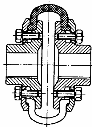
6-12. Periflex tengelykapcsoló
