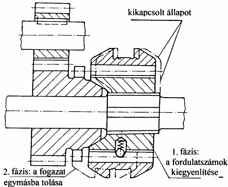
6-16. ábra. A szinkronizáló szerkezet elvi vázlata
