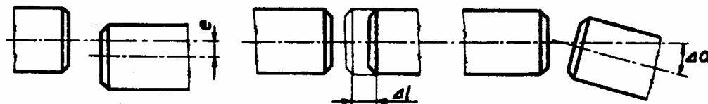
6-4. ábra. Tengelyek helyzeteltérései
