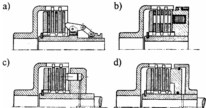
6-18. ábra. A kapcsolóerő létesítésének módja
