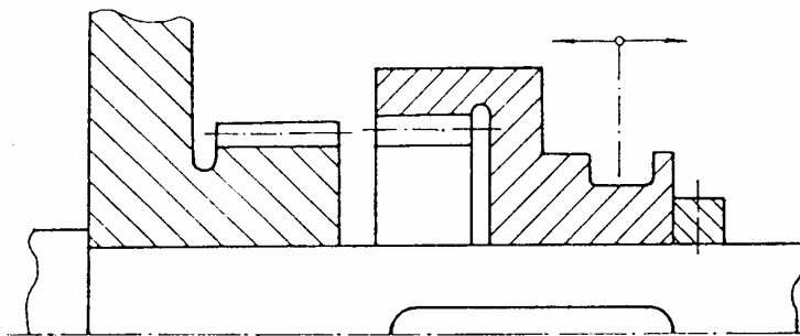
6-15. ábra. A fogazott, oldható tengelykapcsoló vázlata.
