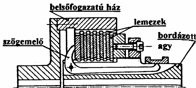
6-20. ábra. Lemezes dörzskapcsoló
