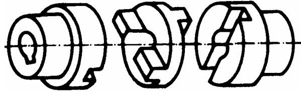
6-5. ábra. Oldham-féle tengelykapcsoló
