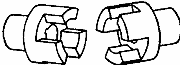
6-6. Körmös tengelykapcsoló.
