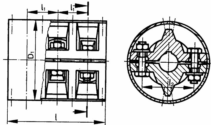
6-2. ábra. Héjas kapcsoló.
