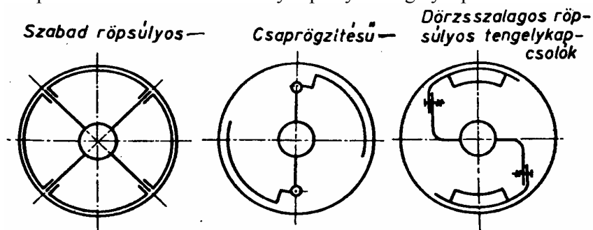
6-25. ábra. Röpsúlyos tengelykapcsolók elvi vázlata.
