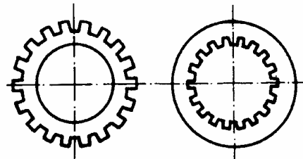
6-21. ábra. Többlemezese dörzskapcsoló kívül és belül fogazott lemezei
