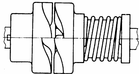
6-26. ábra. Körmös szabadonfutó.
