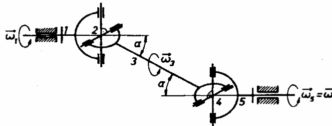
6-9. ábra. Párban alkalmazott kardán kapcsolók.
