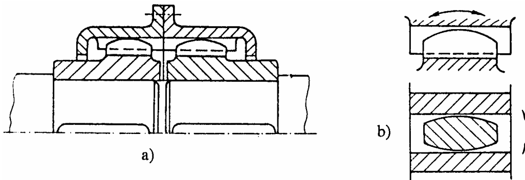
6-7. ábra. Fogasgyűrűs tengelykapcsoló(a); A fogak kialakítása (b).
