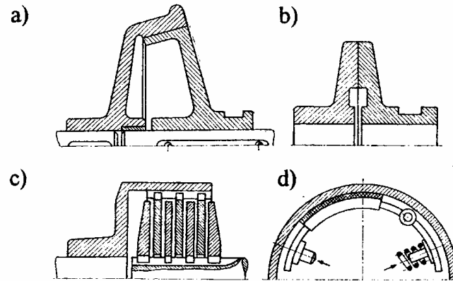
6-17. ábra. Dörzskapcsolók súrlódó felületeinek alakja.
