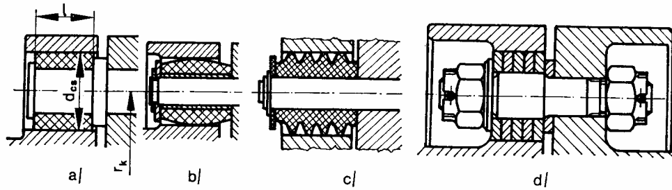
6-11. ábra. Dugóalkalítások.
