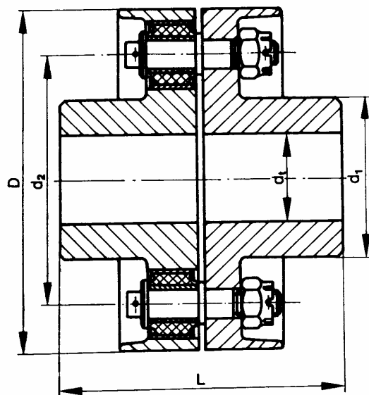
6-10. ábra. Rugalmas, dugós tengelykapcsoló
