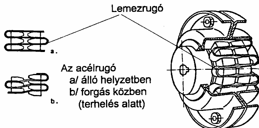
6-13. ábra. Acélszalagos tengelykapcsoló
