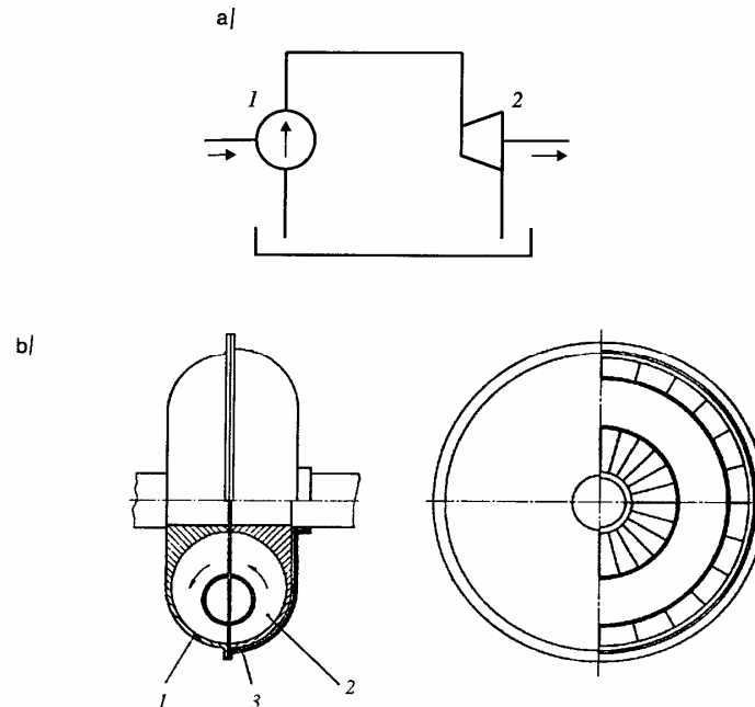
6-23. ábra. Hidrodinamikus tengelykapcsoló működési elve.
