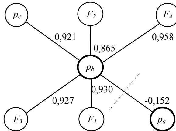
5.4. ábra Korrelációcsalád vizsgálat eredménye
