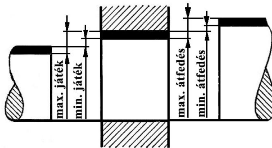
Laza és szoros illesztés
