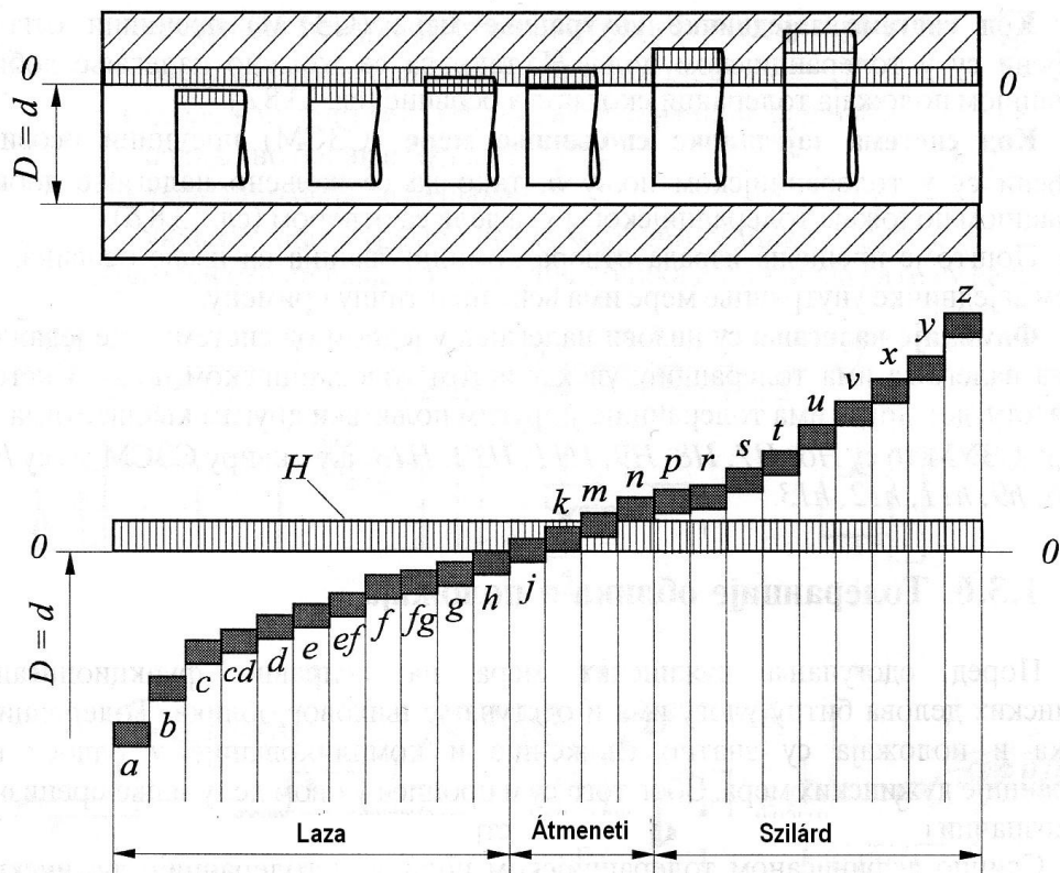
A tűrésmezők elhelyezkedése az alaplyuk-rendszerben
