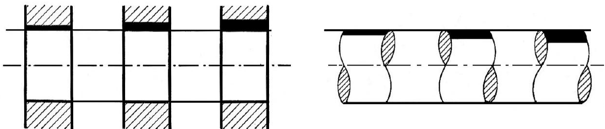
Különböző tűrésmező nagyság furat és csap esetében
