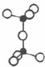
b) [Si_2O_7]^{6-}
