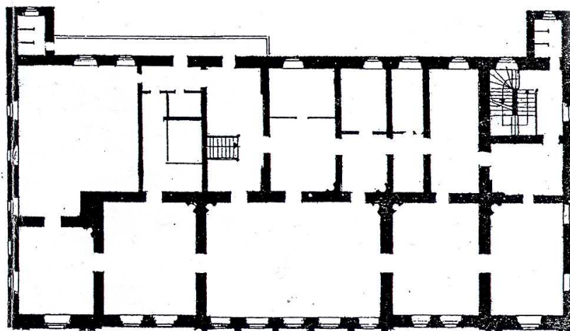
32. A Kendeffy-ház földszinti alaprajza
