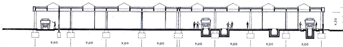
135c ábra. Budapest III., Rádl-ároki gépjárműtelep metszete
