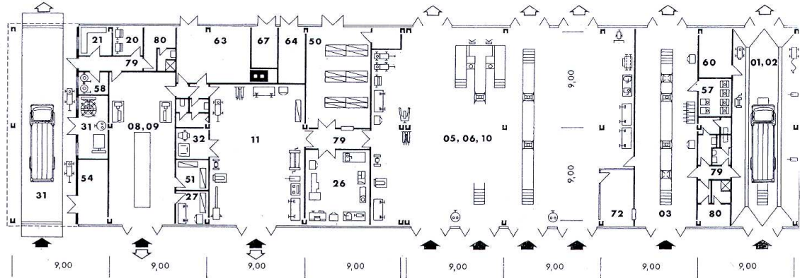
135b ábra. Budapest III., Rádl-ároki gépjárműtelep alaprajza
