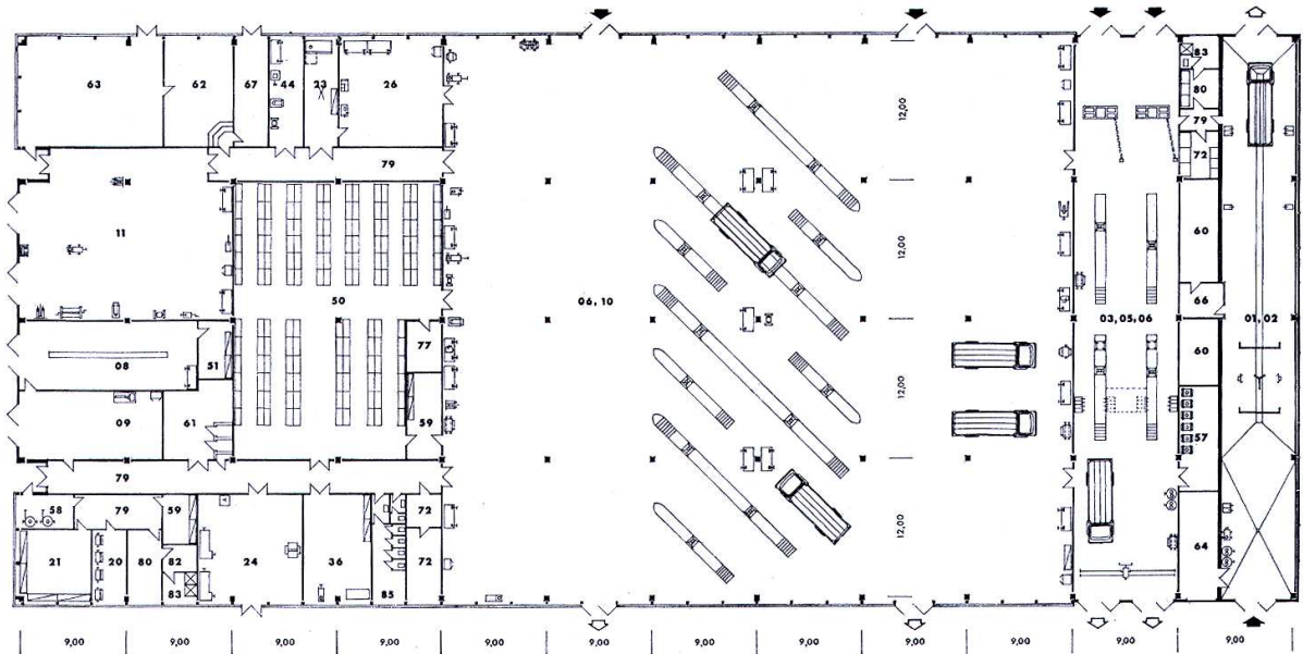
147b ábra. Budapest IX., Illatos úti gépjárműtelep, üzemi épület alaprajza
