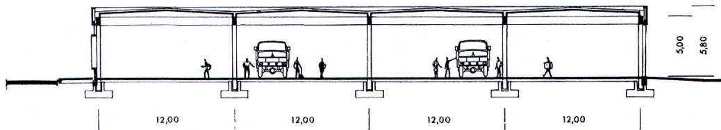
147c ábra. Budapest IX., Illatos úti gépjárműtelep, üzemi épület metszete
