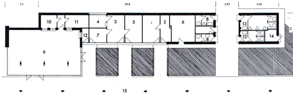
63. ábra. A szombathelyi autóbuszállomás alaprajza
