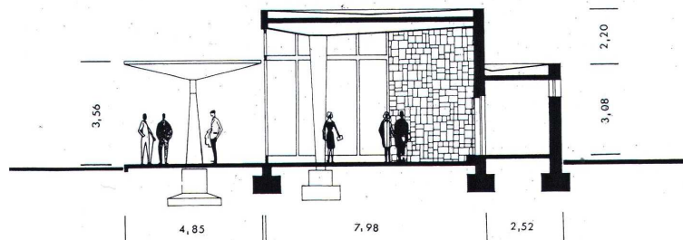
65. ábra. A szombathelyi autóbuszállomás metszete
