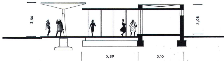
64. ábra. A szombathelyi autóbuszállomás metszete
