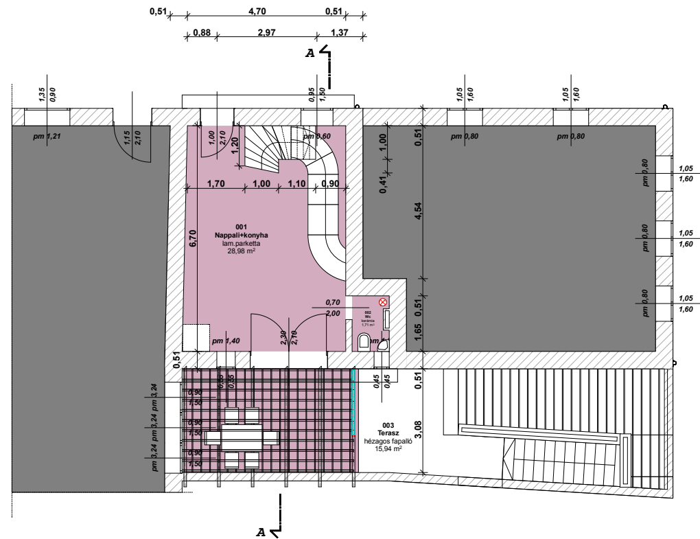
FÖLDSZINTI ALAPRAJZ
