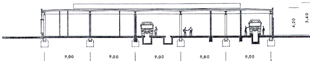
134c ábra. Oroszlány, Táncsics utcai gépjárműtelep metszete
