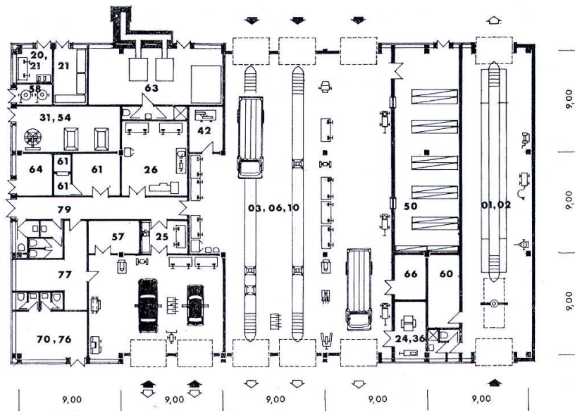
134b ábra. Oroszlány, Táncsics utcai gépjárműtelep alaprajza
