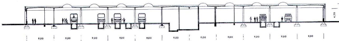
138c ábra. Vác, Deákvári körúti gépjárműtelep metszete
