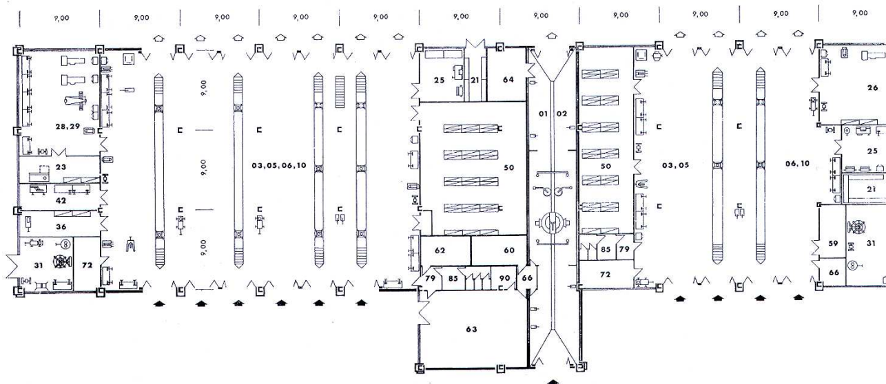
138b ábra. Vác, Deákvári körúti gépjárműtelep alaprajza
