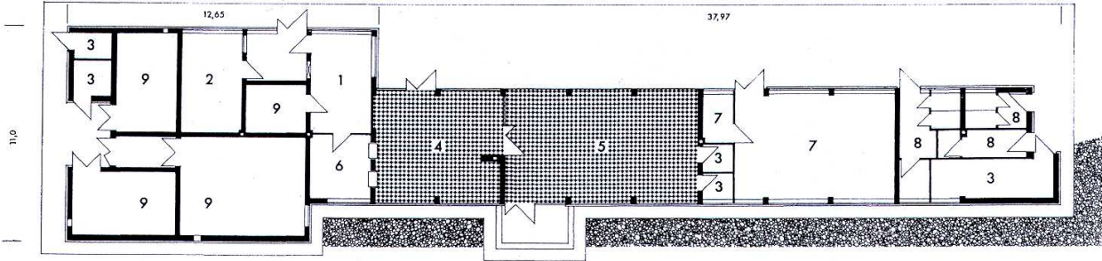
150. ábra. A badacsonytomaji vasútállomás alaprajza
