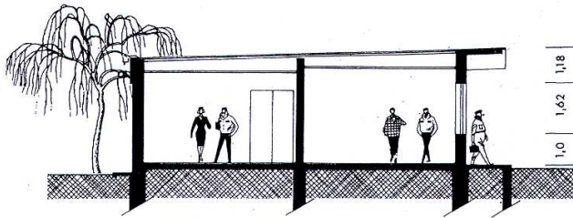
151. ábra. A badacsonytomaji vasútállomás keresztmetszete
