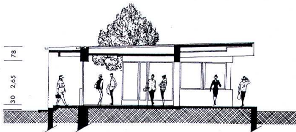
152. ábra. A badacsonytomaji vasútállomás keresztmetszete
