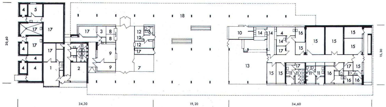
146. ábra. Az alsóörsi vasútállomás alaprajza
