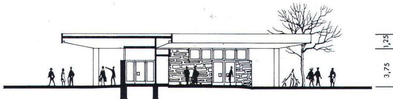
147. ábra. Az alsóörsi vasútállomás keresztmetszete
