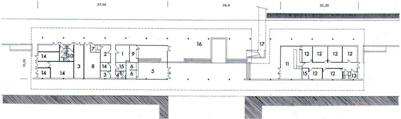
159. ábra. A balatonfenyvesi vasútállomás alaprajza
