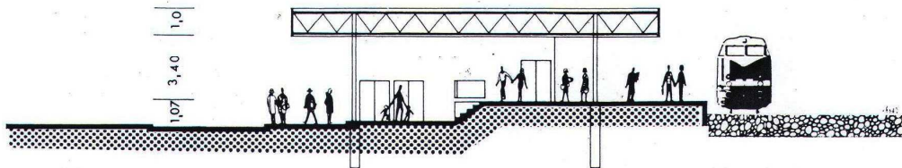
160. ábra. A balatonfenyvesi vasútállomás keresztmetszete
