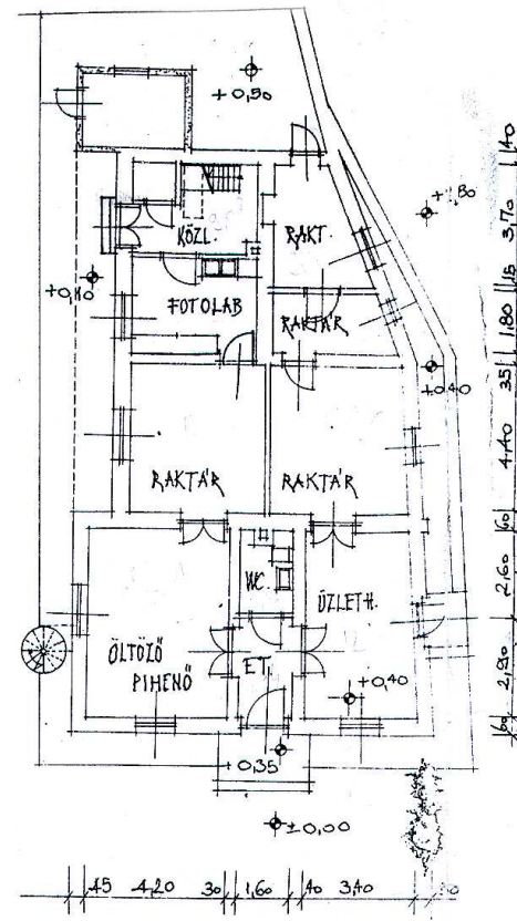
FÖLDSZINTI ALAPRAJZ M-1:200
