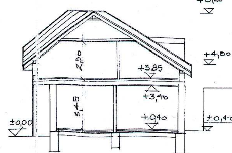
METSZET M-1:200
