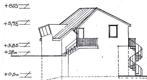
NYUGATI HOMLOKZAT M-1:200
