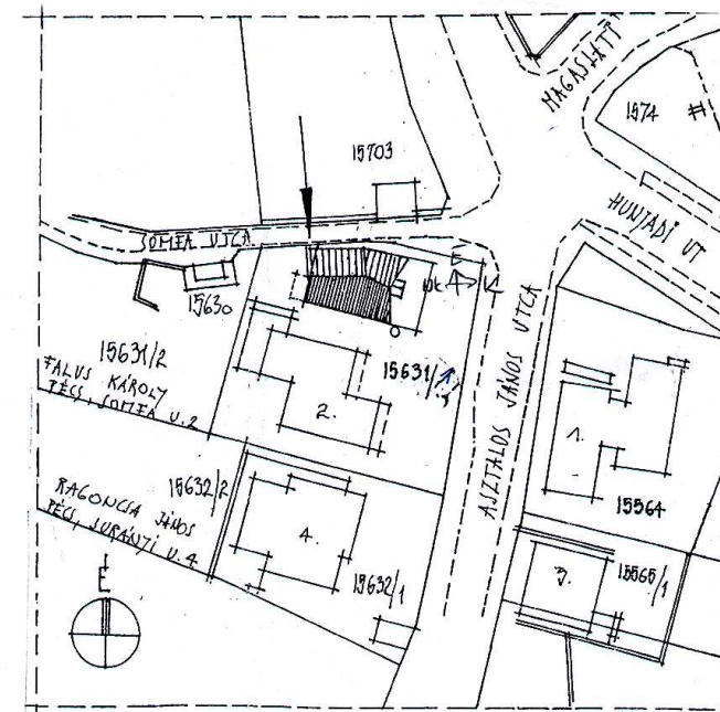
HELYSZINRAJZ M-1:1000
