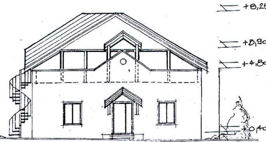
KELETI HOMLOKZAT M-1:200
