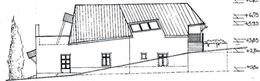
ÉSZAKI HOMLOKZAT M-1:200
