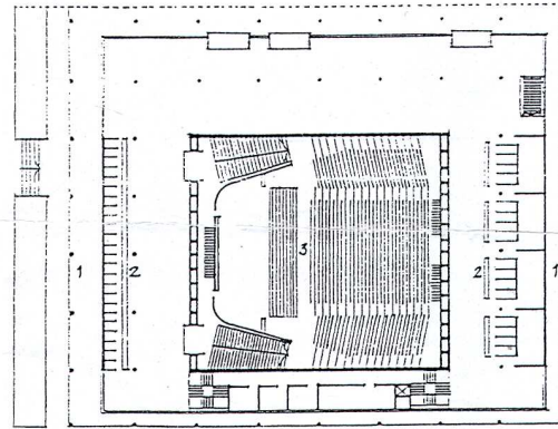
A HAGYÓDÓTEREM ALAPRAJZA 914 ÜLŐHELY
