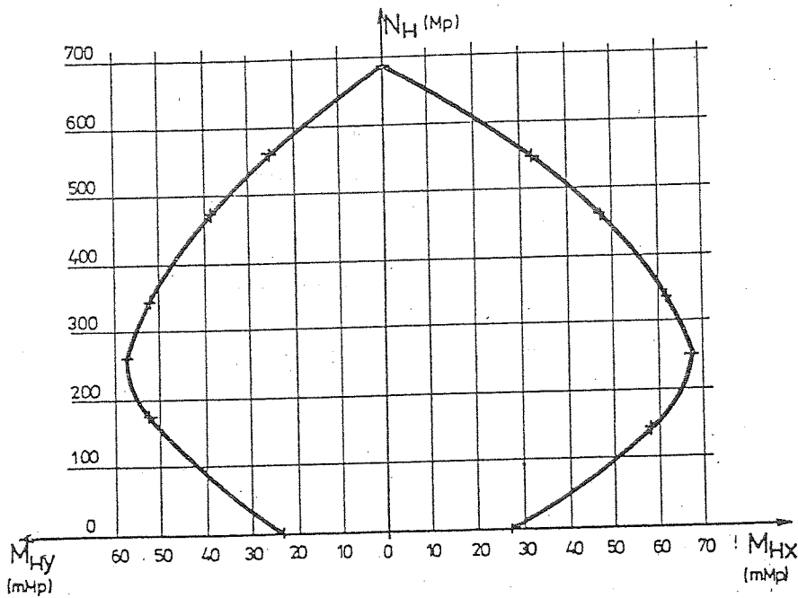
Tegerbirás (befogás keresztmetszetében)
