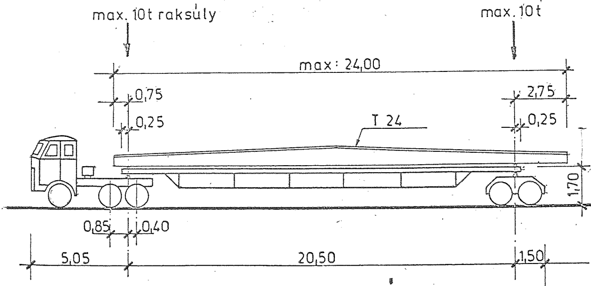
IKERTENGELYES MAZ NHE-24
