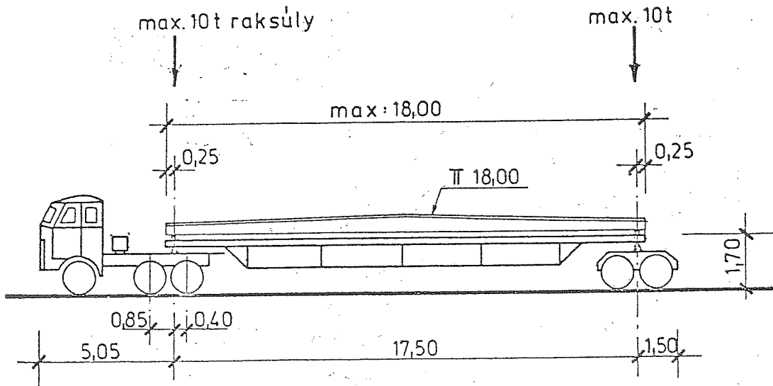
IKERTENGELYES MAZ NHE-18
