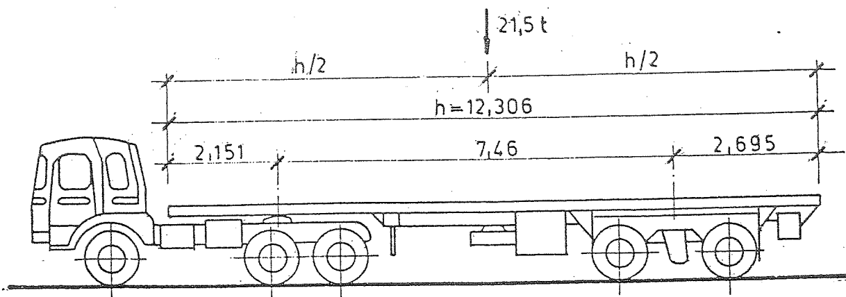
RABA 576
