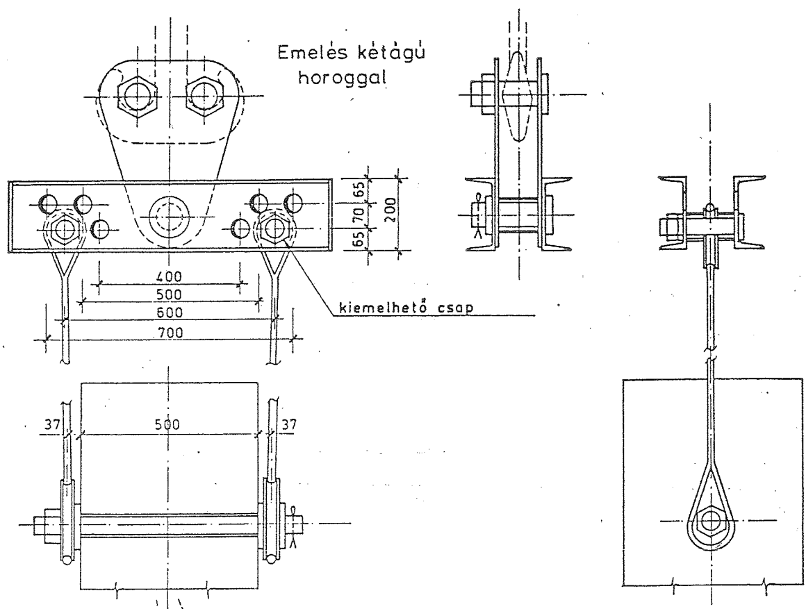
Emelés egyágú horoggal
