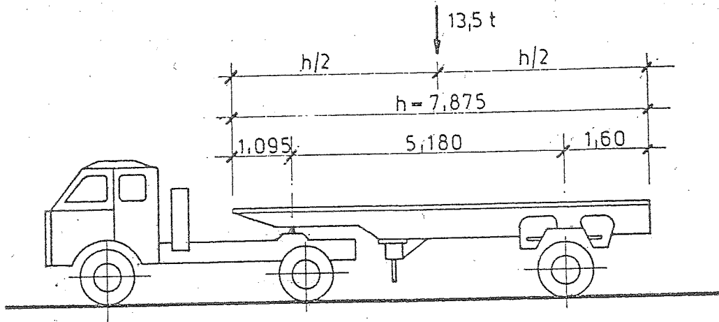
MAZ 5245
