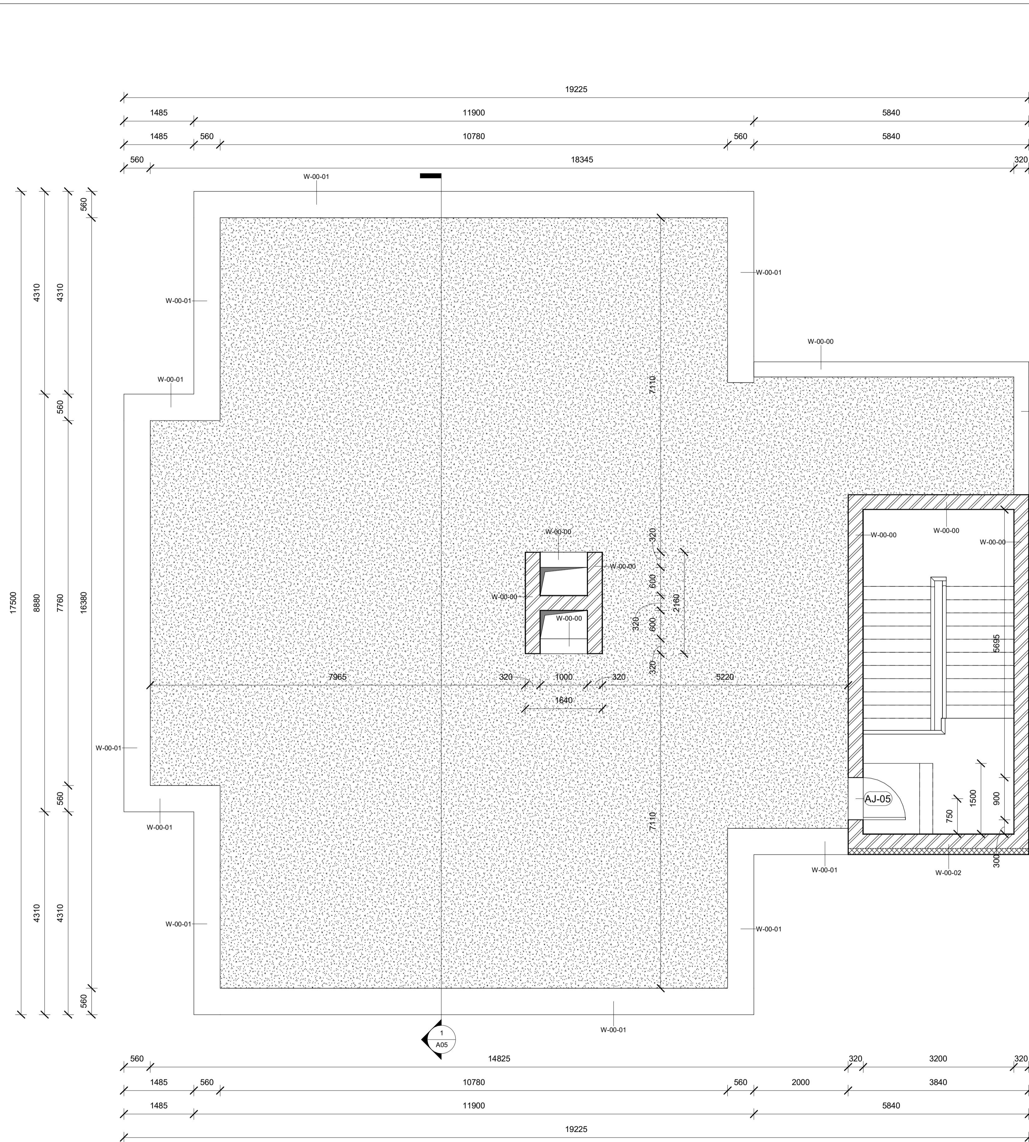
1 04 Tető 1 : 50
