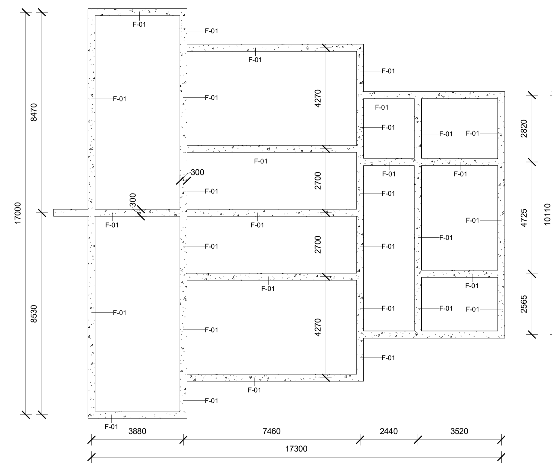
2 A1 Alapozás felső síkja 1 : 100
