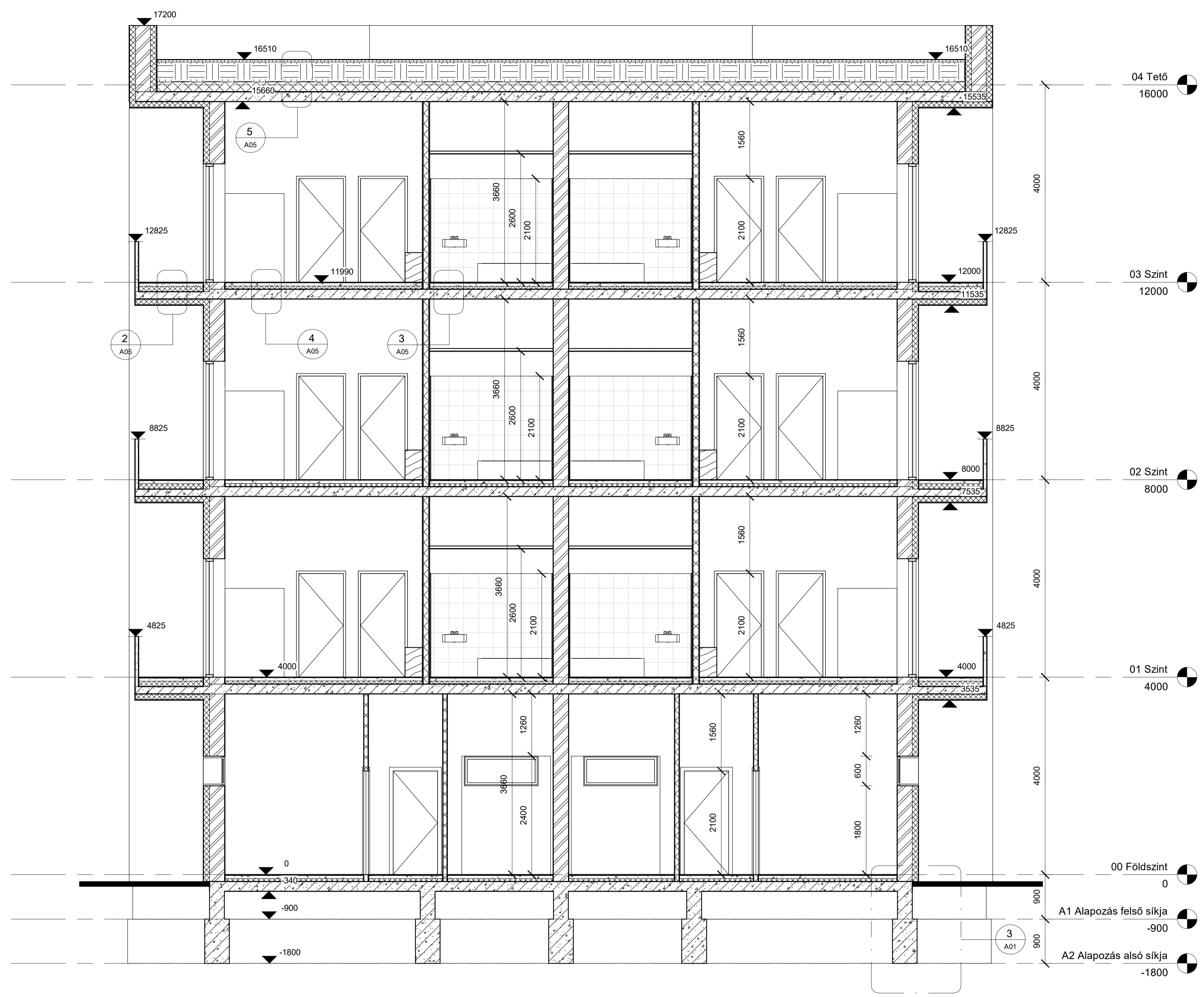
1 Metszet 1 1 : 50
