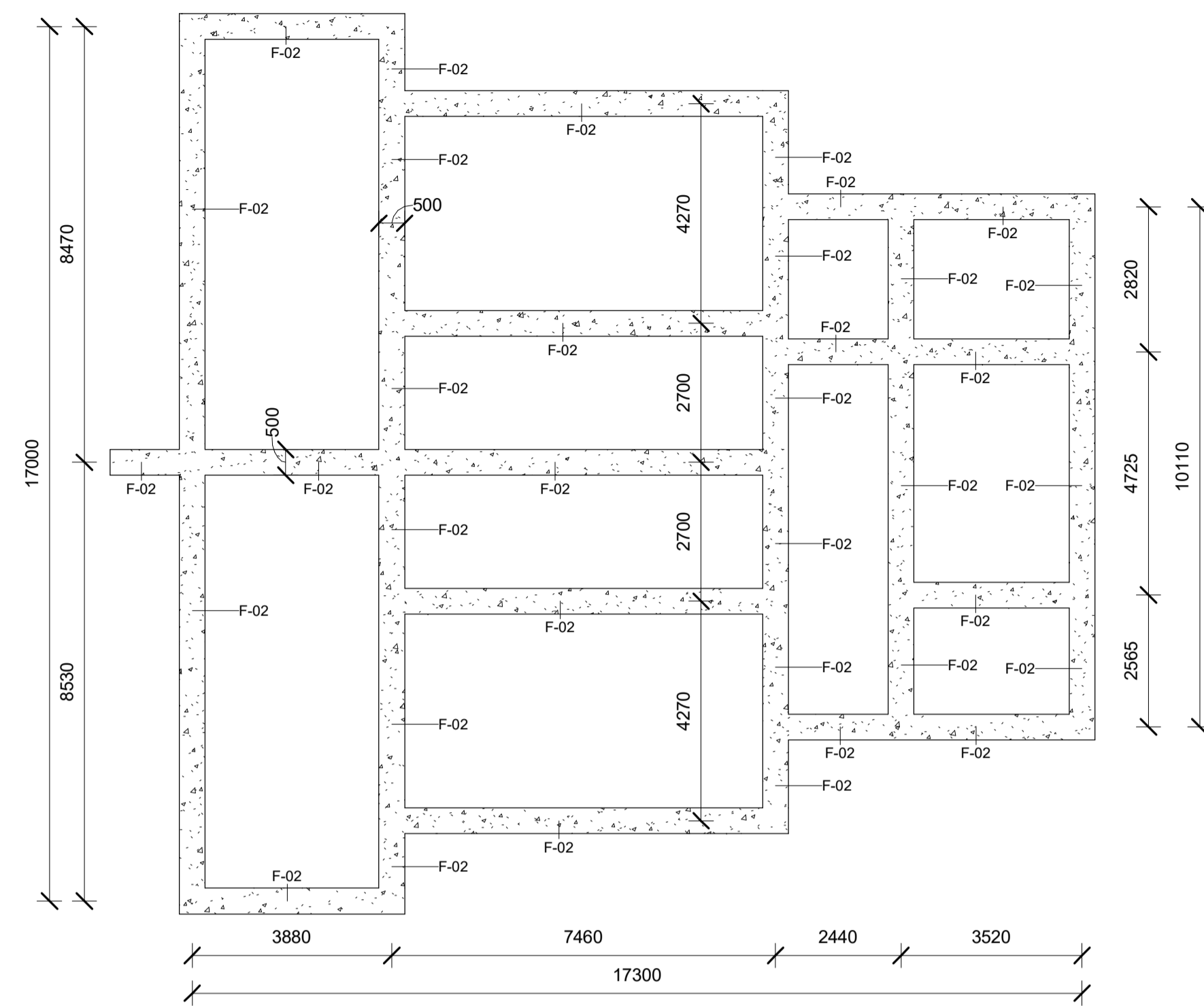
1 A2 Alapozás alsó síkja 1 : 100
