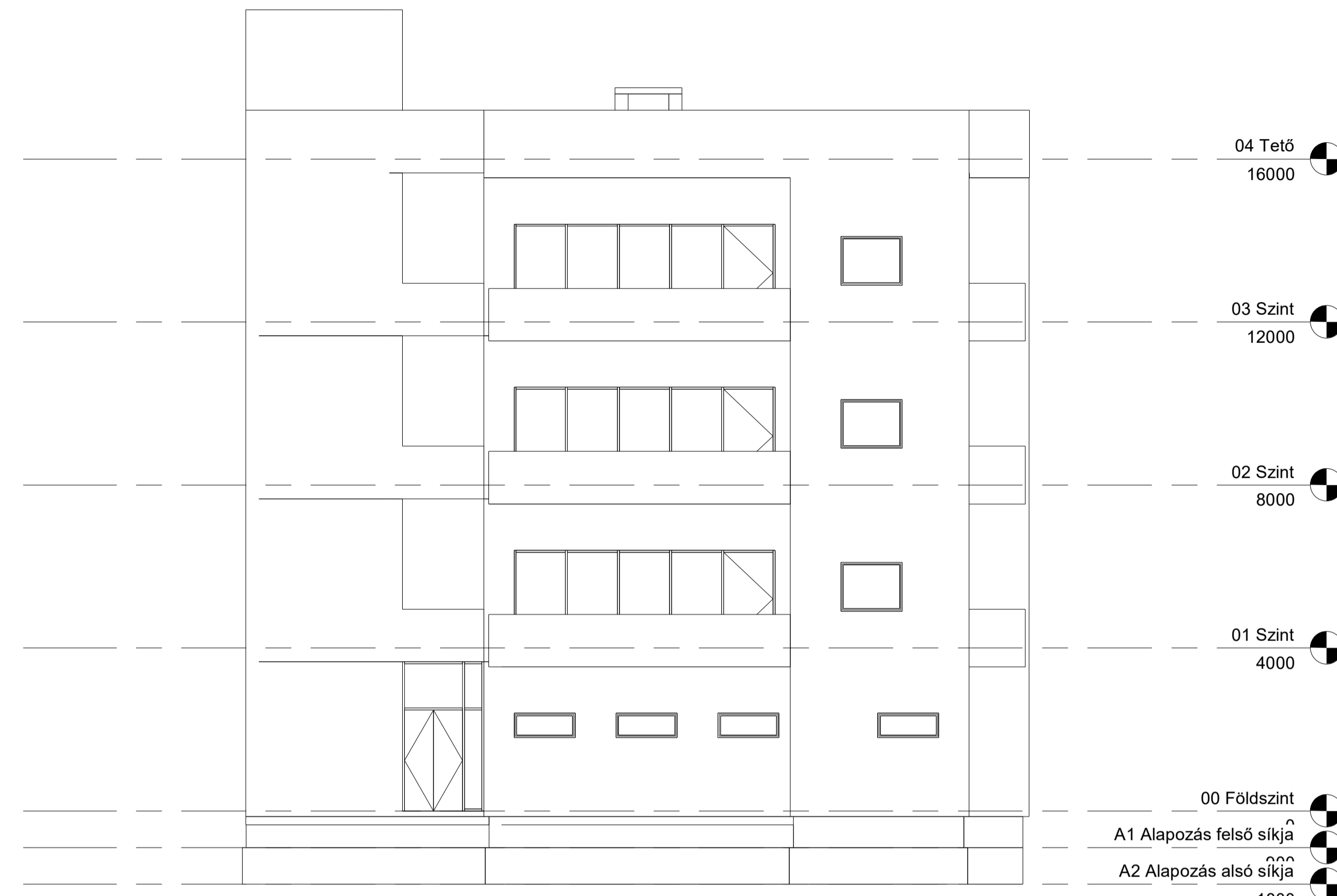
2 North 1 : 100
