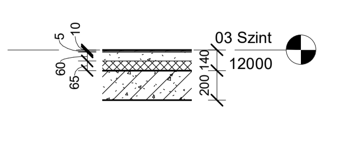
4 Részlet 3 1 : 25
