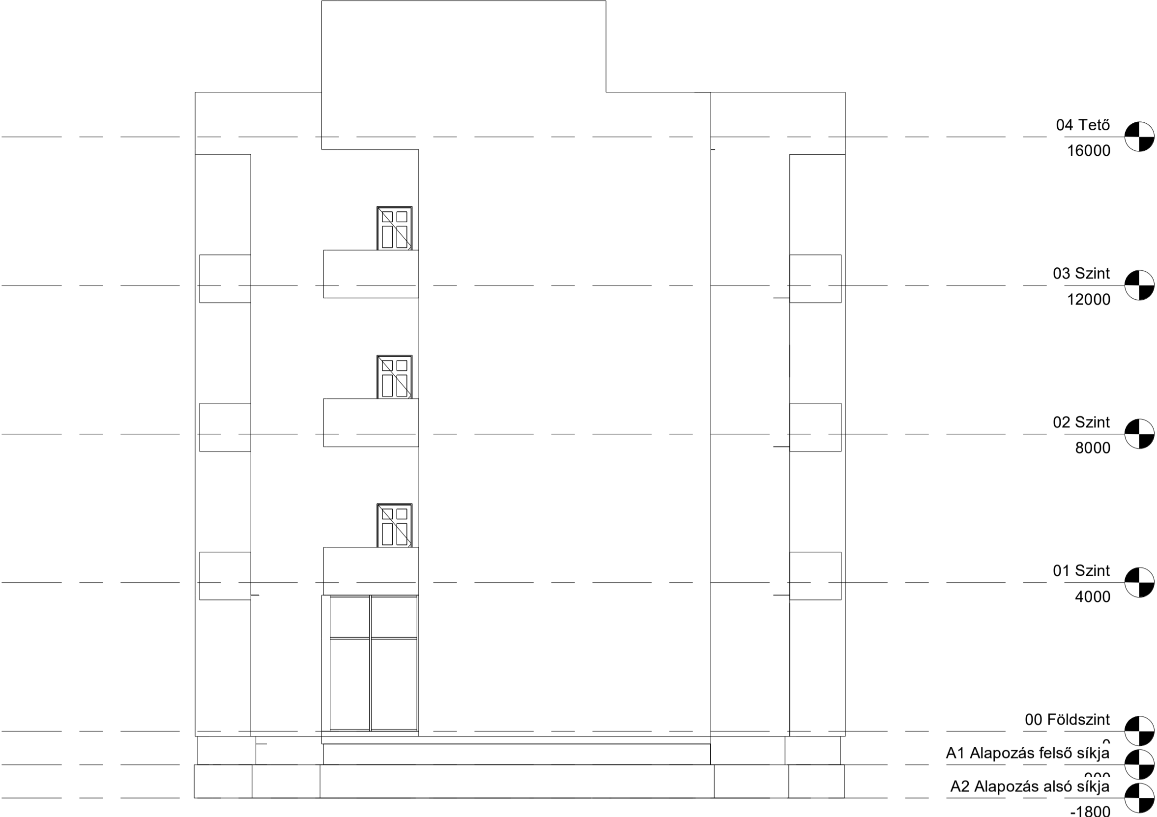
1 East 1 : 100
