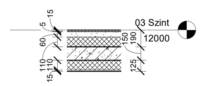
2 Részlet 1 1 : 25
