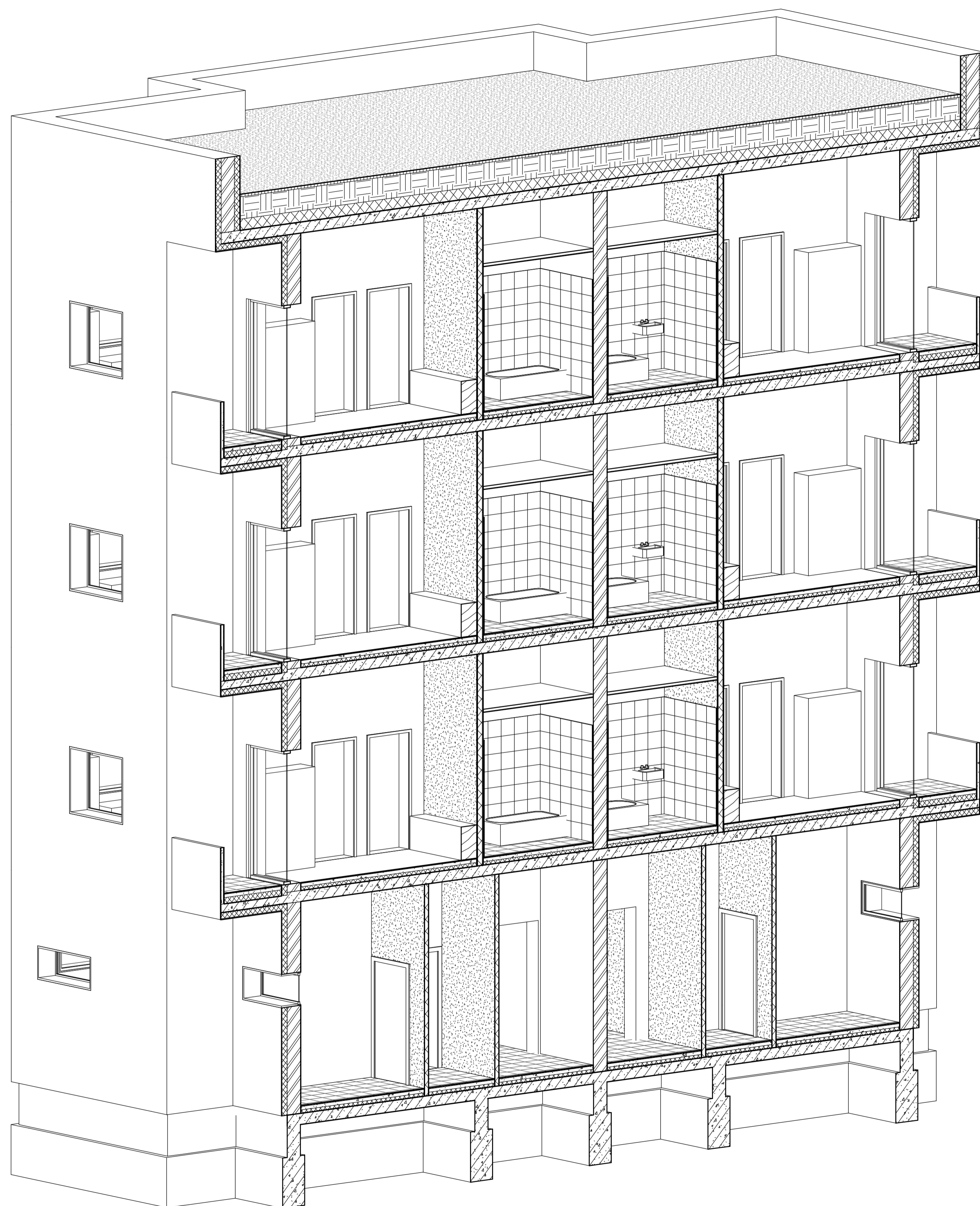
1 3D Metszet
