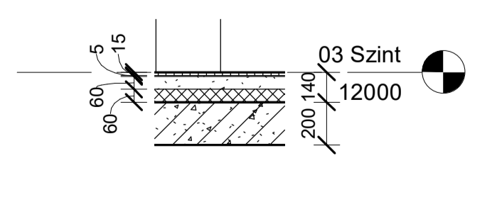
3 Részlet 2 1 : 25
