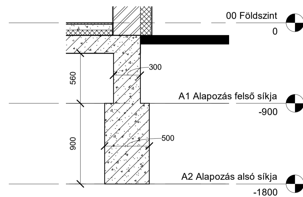
3 Alapozás 1 : 25
