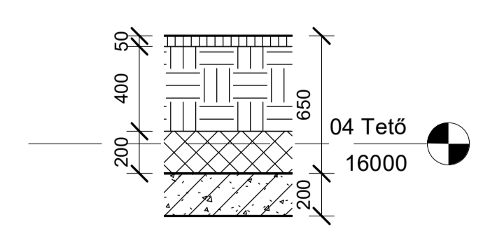
5 Részlet 4 1 : 25
