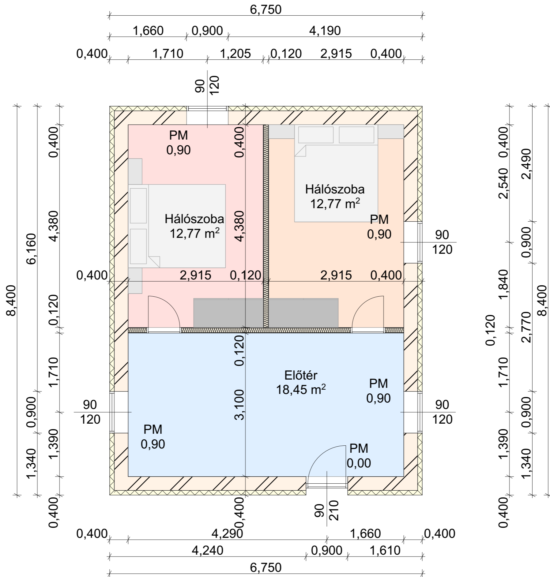
Alaprajz 1:50
