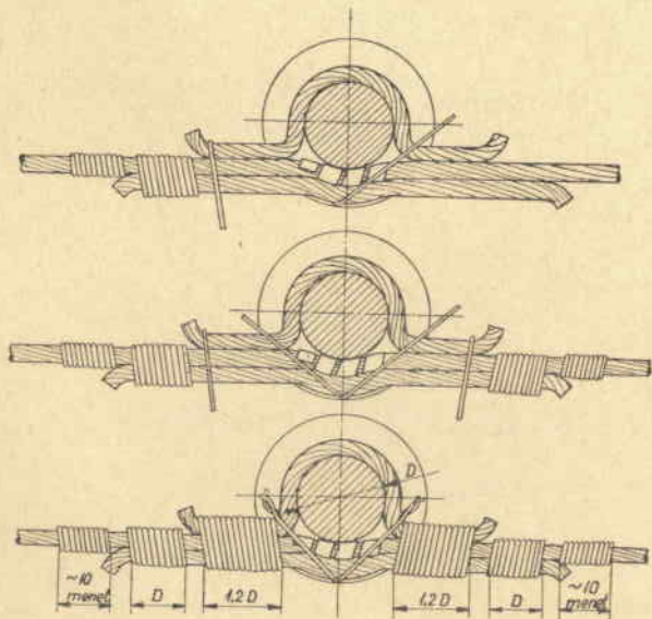
49. ábra. Csillapító kengyeles kötés
