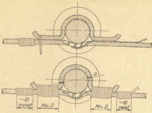
48. ábra. Kengyeles kötés
