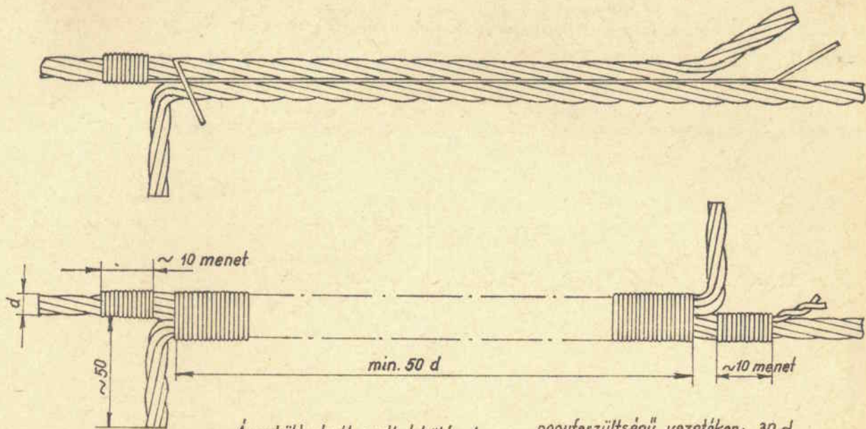
51. ábra. Pólyás toldókötés
