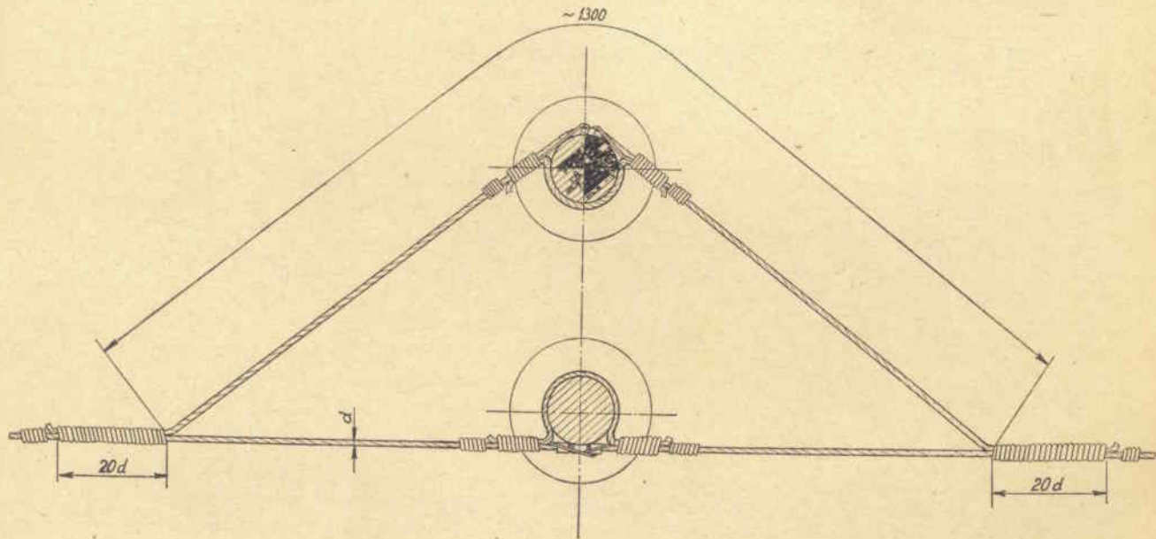
50. ábra. Tartókötés két szigetelőn kengyeles kötéssel
