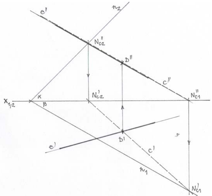
1/2. Szerkesztés menete: A II. ks.-ban az e egyenes
