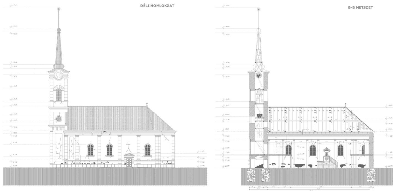
Református templom kárfelmérési építészeti tervei (Forrás: dr. Horváth M., Turi T.)
