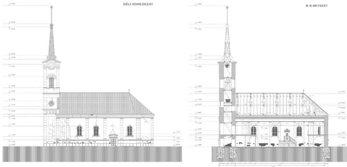
Dr. Horváth M., Turi Tamás: Dunaszentgyörgyi református templom épülete – épületfelmérés, épületdiagnosztika
